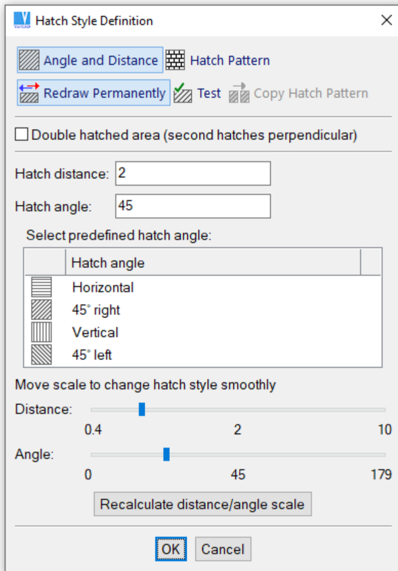
Seleção de Padrão Simples
