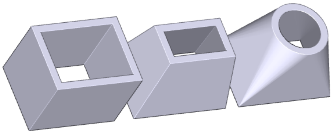
Exemplo de extrusão, loft prismático e loft de um retângulo para um círculo
