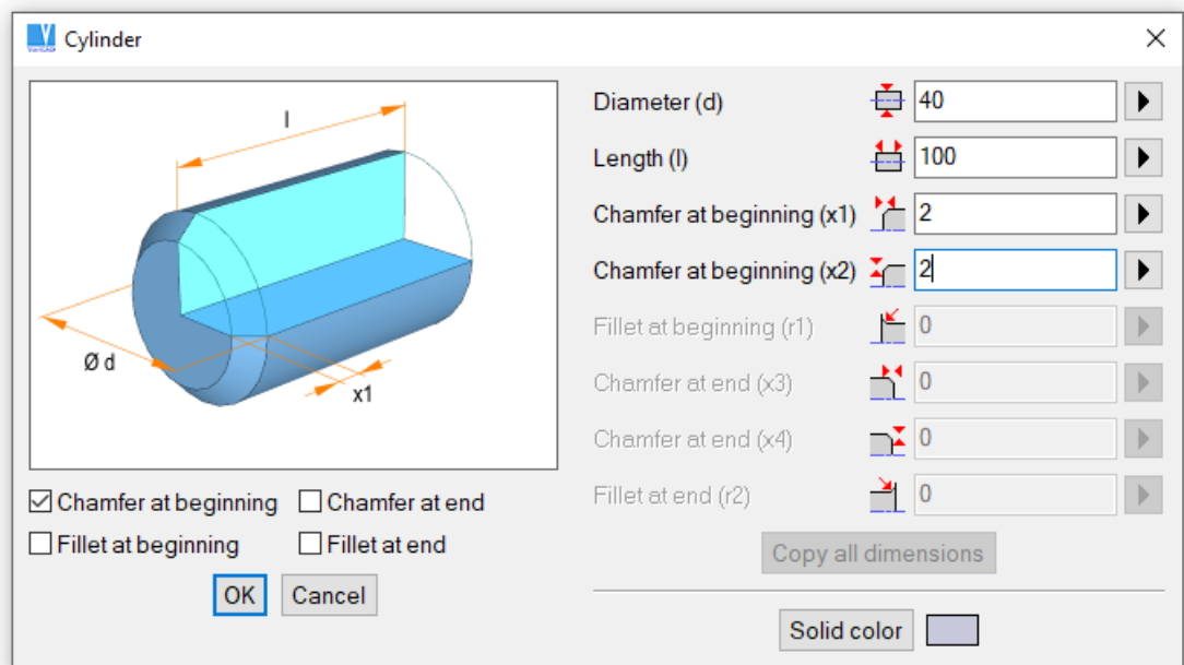
Exemplo de definição da forma e dimensões de um cilindro
