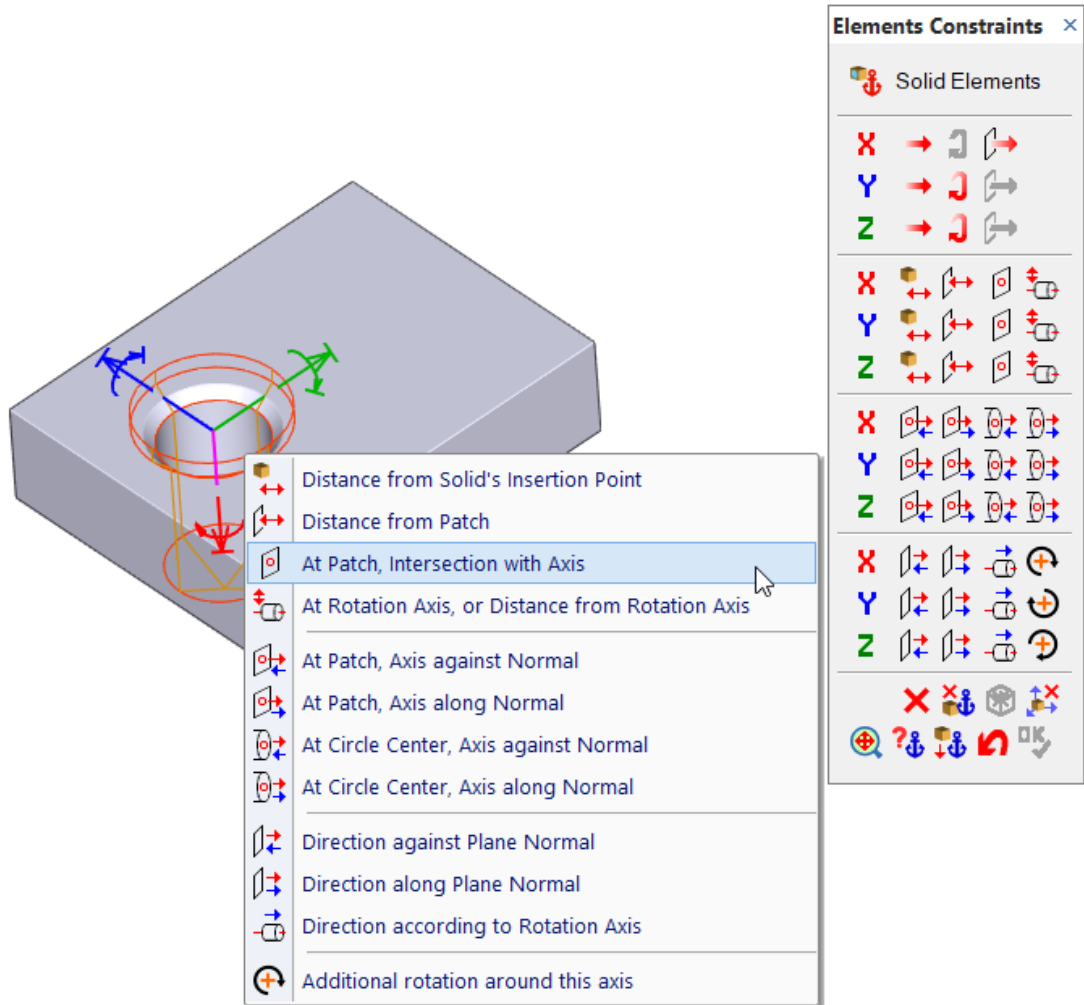
Definição de constrangimentos, Painel de constrangimentos
