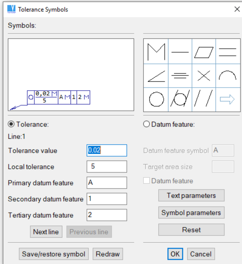
Definição dos símbolos de tolerância
